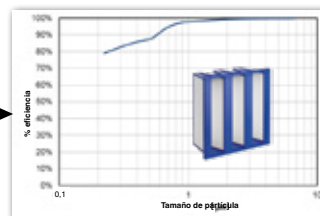
2ª etapa filtrante Filtro ePM1 85% (F9)
