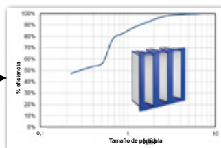
1ª etapa filtrante Filtro ePM1 55% (F7)
