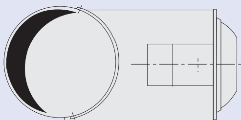
Exemple de raccordement sur gaine circulaire
