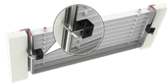
Fixation par vis dissimulées sans contre-cadre
